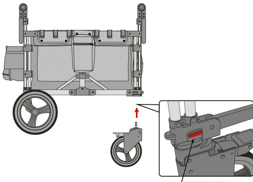
Botón de liberación rápida de la rueda delantera
