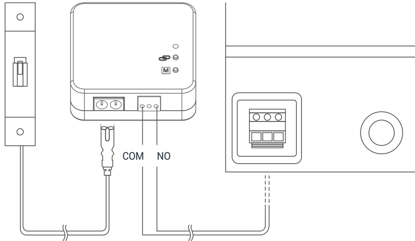
Σχέδιο σύνδεσης
