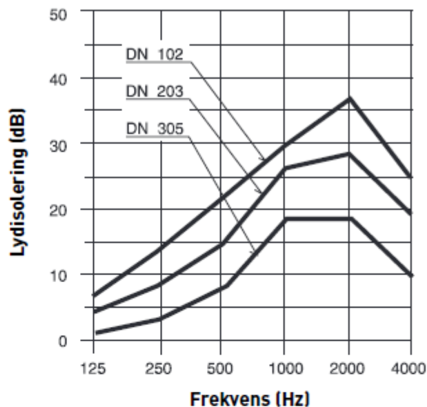
Diagram 2: Lydniveau Isoleringstykkelse: 25 mm Rørlængde: 1000 mm
