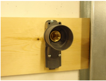
Gipsdåse Monteret på bræt påsat rekler.
