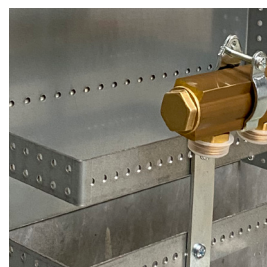
Max. bestykning af et BUNDMODUL for at det kan være i et 60 cm skab. 12 GV, 16KV og 9VV.
