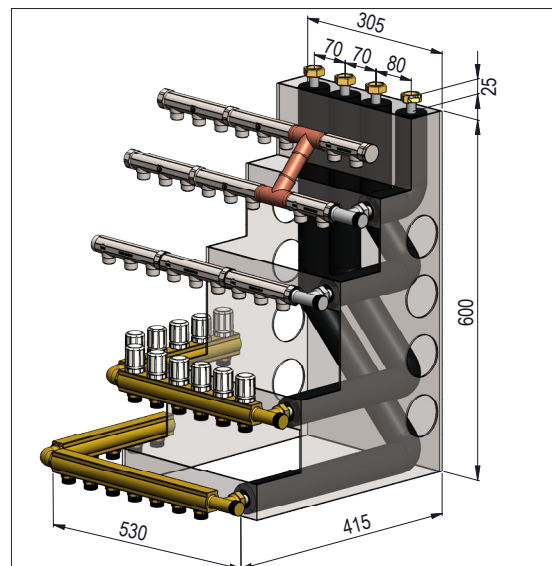
Max. bestykning af et BUNDMODUL for at det kan være i et 60 cm skab. 12 GV, 16KV og 9VV.
