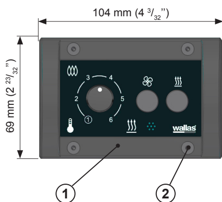
Koppla styrpanelens ledning från apparaten till styrpanelen (1). Sätt fast styrpanelen i installeringsöppningen med festsättningskruvar (2).
