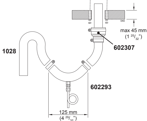
Installation av förslutbar däckgenomföring 2466. Monteringshålet ska vara \varnothing 50 mm (2") och skruvhålen 4 x 6 mm.
