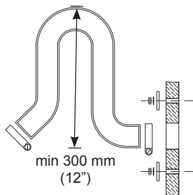
Zwanenhals
