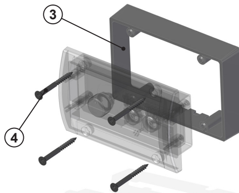
Vid ytinstantiering av styrpanelen används halsen/kanten (3). I paketet medkommer 4 st festsättningskruvar, 3,5 x 40 mm (svart) TX 10 (4).
