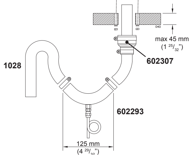
Installatie van de afsluitbare dakuitlaat 2466 . Het installatie gat is \varnothing 50 mm en de gaten van de schroeven 4 x 6 mm.
