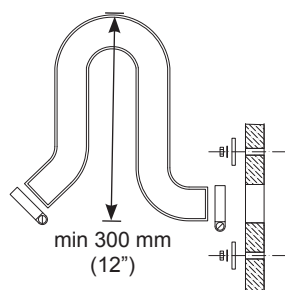
Svanehals
