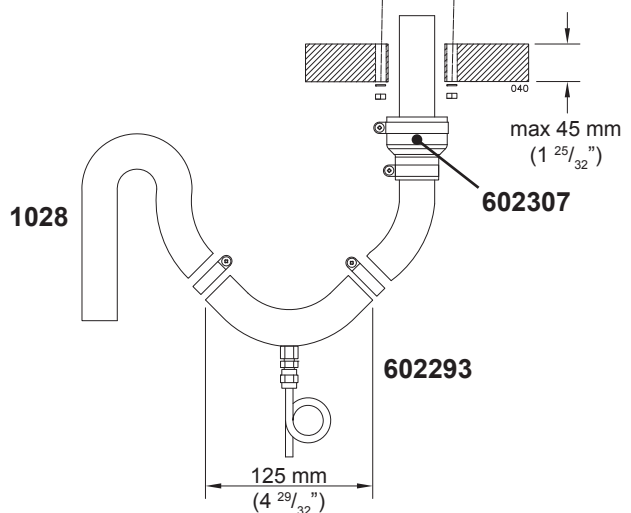
Installasjon av forseglbar dekkgjennomføring 2466 . Installasjonshullet er \varnothing 50 mm skruehuller 4 x 6 mm.
