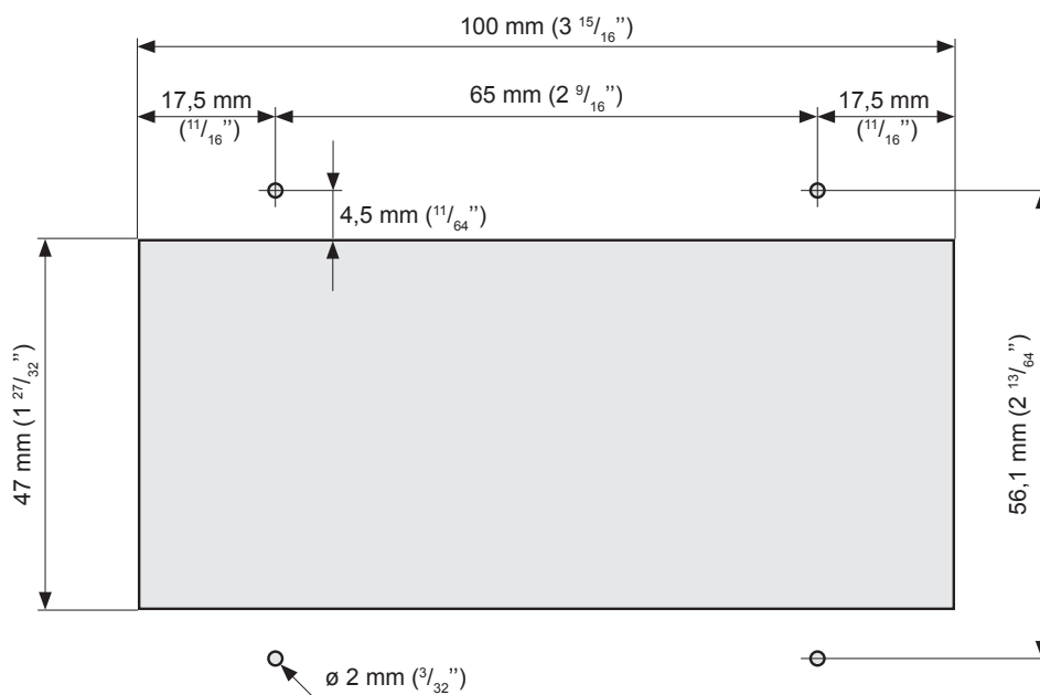
Måttet på kontrollpanelens installeringsutrymme Förborra vid behov hål för de 2 mm (3/32") skruvarna.
