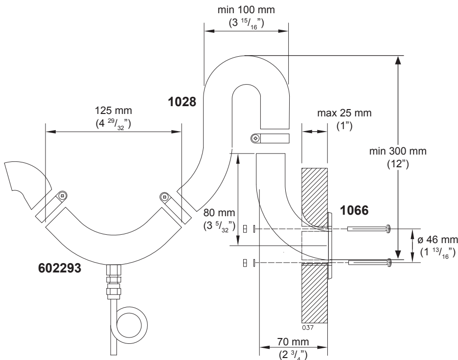
Installation der Abgasdurchführung 1066 im Rumpf. Die Installationsöffnung beträgt \varnothing 35 \text{ mm} ( 1 \frac{3}{8} " ) und die Schraubenbohrungen sind 4 \times \varnothing 5 \text{ mm} .
