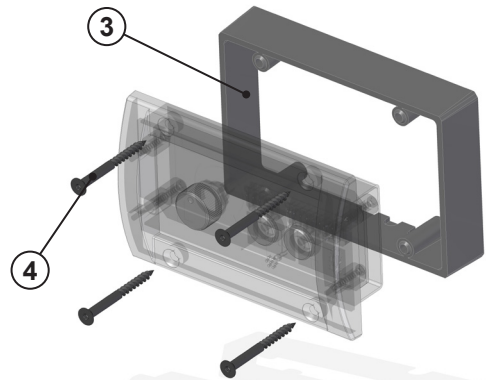
Ohjauspaneelin pinta-asennukseen käytetään pinta-asennus kaulusta (3). Pakkauksen mukana tulee kiinnitysruuvit 4 kpl 3,5 x 40 mm (musta) TX10 (4).
