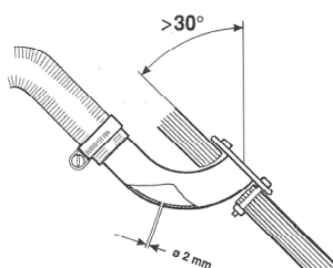
Peräpeiliin asennus
