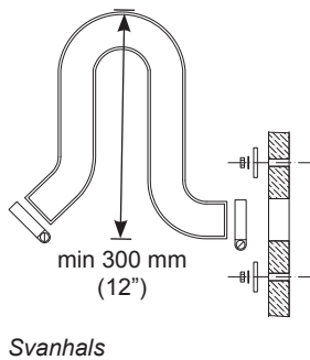
Svanhals
