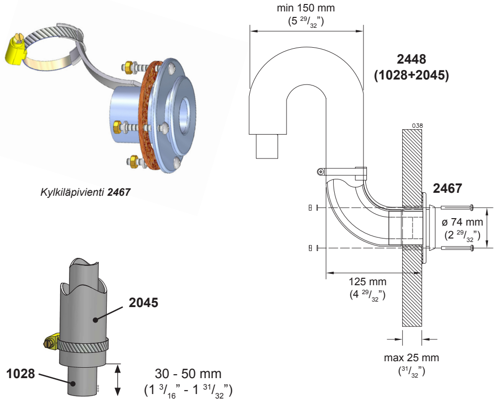
Putkien pituusero
