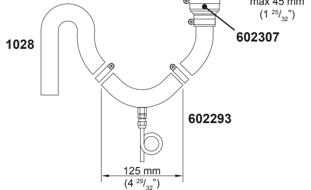
Suljettava kansiläpivienti 2466 asennus. Asennusaukko on \varnothing 50 mm ja ruuvien reiät 4 x \varnothing 6 mm.
