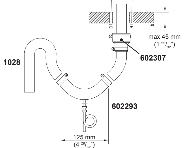
Installation der siegelbaren Deckendurchführung 2466 . Die Installationsöffnung beträgt \varnothing 50 \text{ mm} ( 2 " ) und die Schraubenbohrungen 4 \times 6 \text{ mm} .
