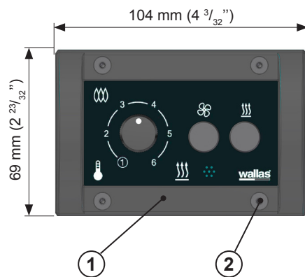
Kytke ohjauspaneelin johto laitteelta ohjauspaneeliin (1). Kiinnitä ohjauspaneeli asennusaukoon kiinnitysruuveilla 4 kpl 3,5 x 20 mm (musta) TX10 (2).
