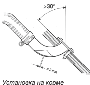
Установка на корме
