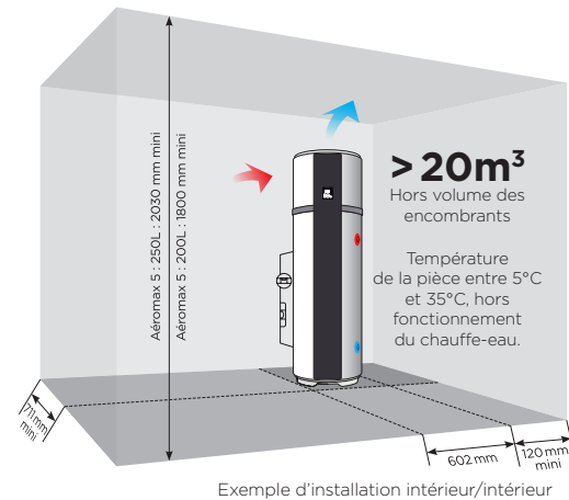
Exemple d'installation intérieur/intérieur
