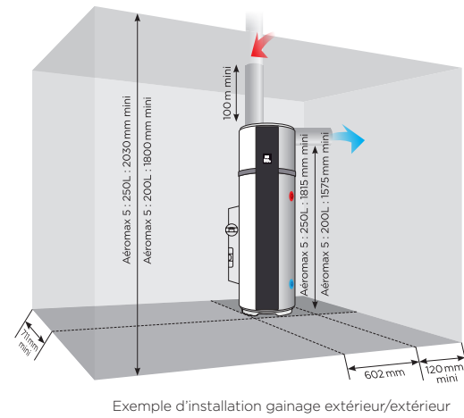
Exemple d'installation gainage extérieur/extérieur
