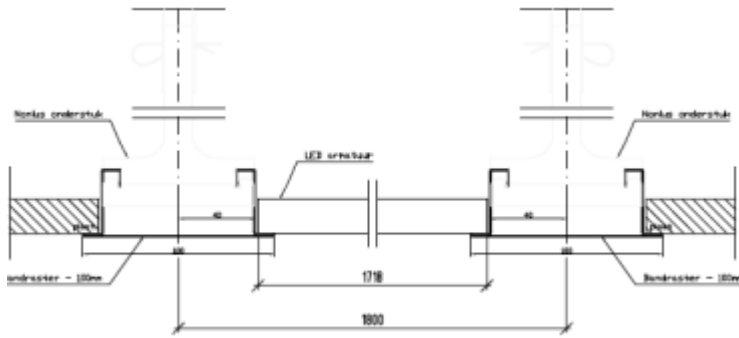
Doorsnede A
