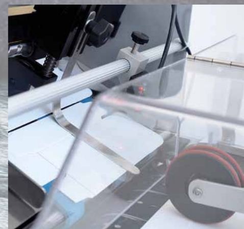
Führungsrad hält das Produkt auf dem Förderband an der richtigen Stelle.
