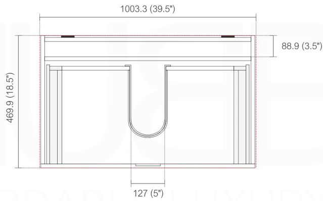
. TOP ELEVATION
