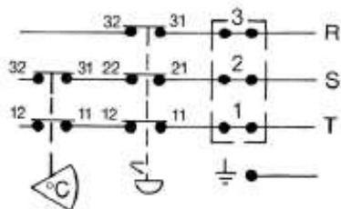
Elschema
