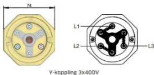
Y-koppling 3x400V
