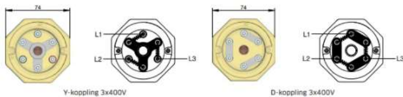
Kopplingschema / inkopplingsalternativ
