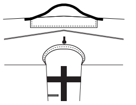
-9- Une fois la boucle ressortie, remplacez le bout présent à l'origine sur la boucle afin de la verrouiller. Puis, remontez la REACTOR Valve.
