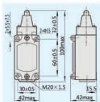
YBLX-K3 Dimensions
