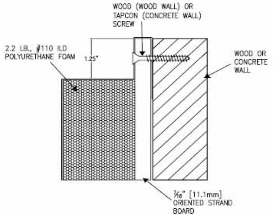
Model 53-1 Wall Padding
