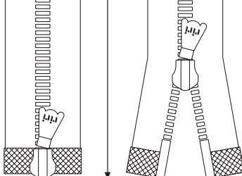
TBCL Two-way open end (Right hand puller, left insert) Divisibile doppio cursore (Apertura a destra, inserimento a sinistra)
