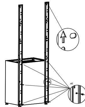
M6 x 16 Screw
