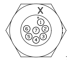
SOLDER LUG VIEW
