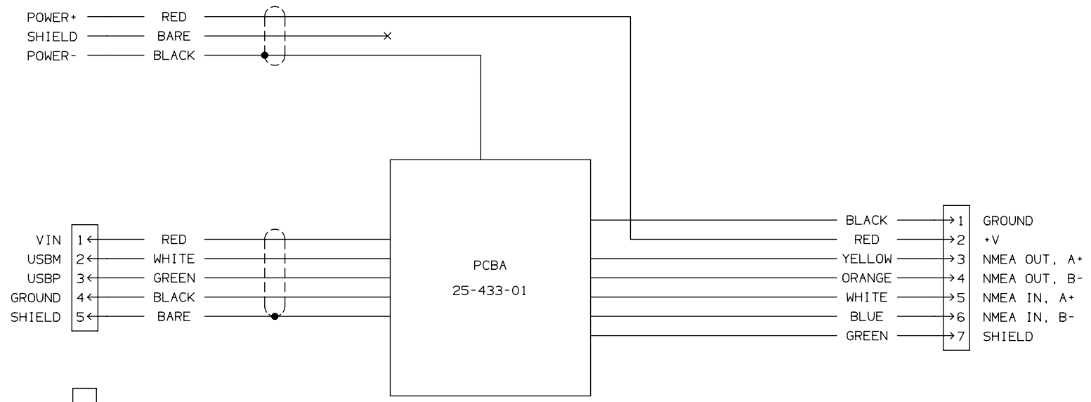
SOLDER LUG VIEW
