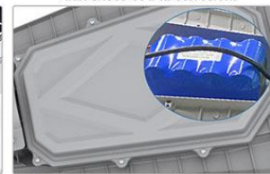
Large batterie intégrée LiFeP04
