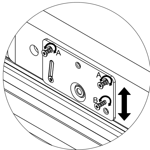
Bottom Roller
