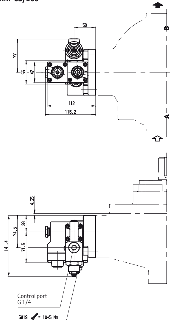
RKP 63/100
