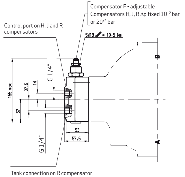
RKP 63/80/100
