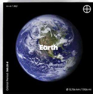
Earth
