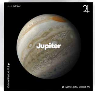
Jupiter
