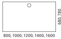
Tischplatte mit Ø80 mm Ausschnitt
