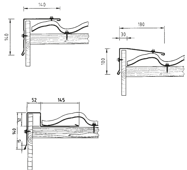
Abb.5 Ortgangausbildung
