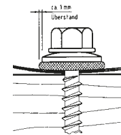
Abb. 3 Befestigung
