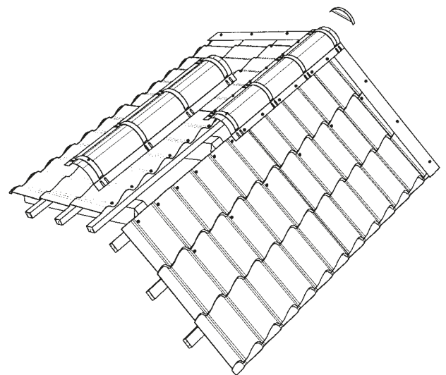
Abb. 6 Montage des Firstes
