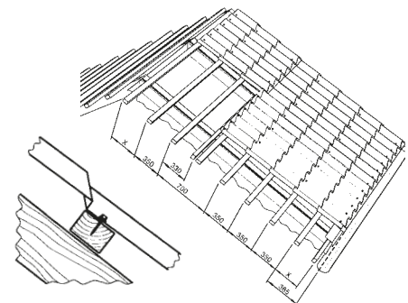
Abb. 1 Lattenanordnung
