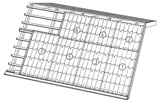
Abb. 4 Montagereihenfolge & Schraubenschema
