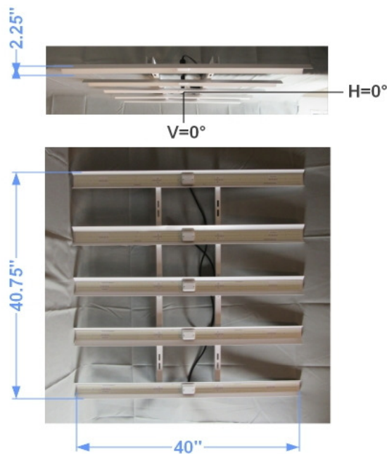
FIG. 1 LUMINAIRE
