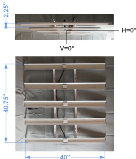
FIG. 1 LUMINAIRE
