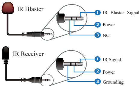
IR BLASTER
