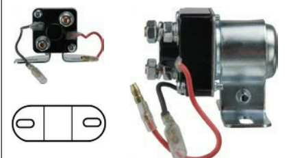
333006 Solenoid
