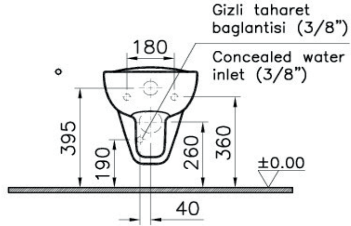
Gizli baglanti Concealed connection versteckte Verbindung
