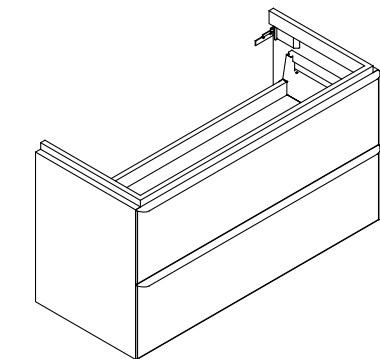
4.1020.2 X. 930 mm Y. 520 mm Z. 410 mm
