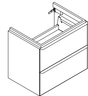
4.1014.2 X. 585 mm Y. 520 mm Z. 410 mm
