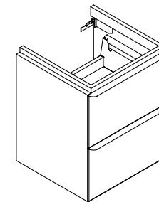
4.1010.2 X. 435 mm Y. 520 mm Z. 410 mm
