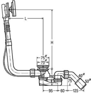
BETTE ABLAUFGARNITUR PLUS 5, Ø 52 mm
