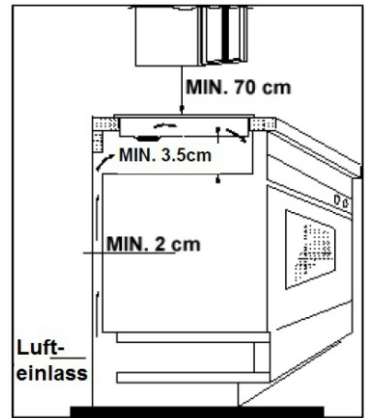
Abbildung 1 Einbau
