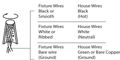
Fig. 2 Wiring
