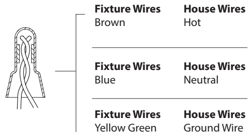
Fig. 2 Wiring
