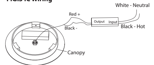
FIG.3 IC Wiring
