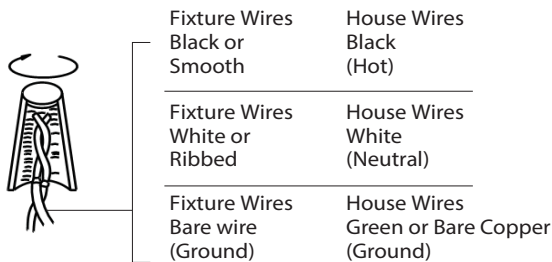
FIG. 2 Wiring
