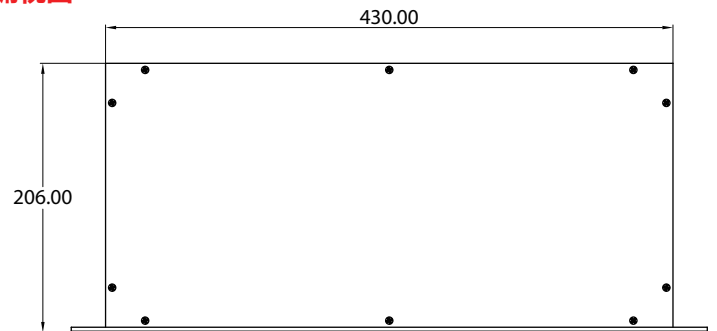
俯视图
