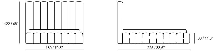
YAT048 / 160 cm - 63''
