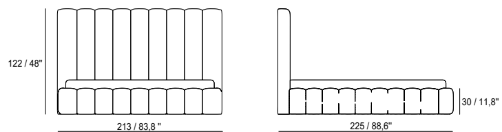
YAT048 / KS
