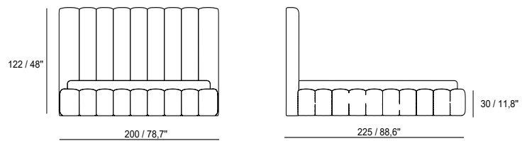
YAT048 / 180 cm - 70,9''
