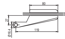
2-teiliges Band CLASSICO 2-part hinge CLASSICO
