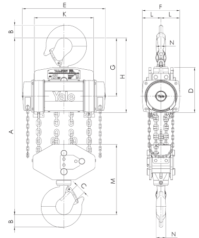
Yalelift 360, 20.000 kg, sechstängig
