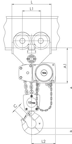
Yalelift ITG, 10.000 kg, dreisträngig
