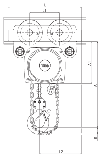
Yalelift ITP/ITG, 500 - 3.000 kg, einsträngig
