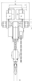
Yalelift ITP/ITG, 5.000 kg, zweisträngig
