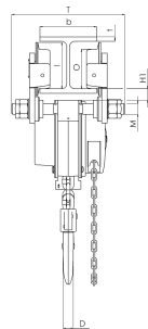
Yalelift ITP/ITG, 500 - 3.000 kg, einsträngig
