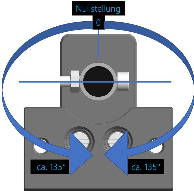
Ansicht von unten auf den OceanMotion
