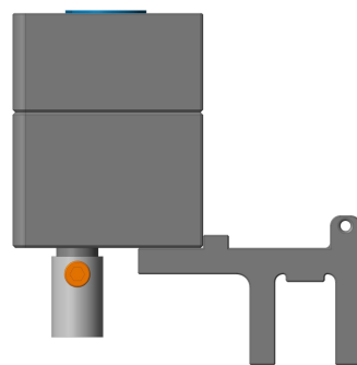
Seitenansicht mit Beckenhalter für Poolbecken
