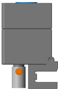
Seitenansicht mit Beckenhalter für Glassteg
