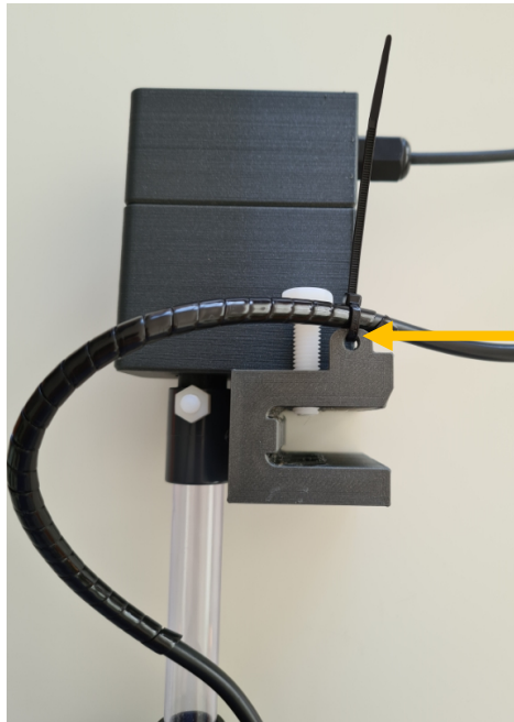
Kabel mit Kabelschutz und fixiert am Beckenrandhalter
