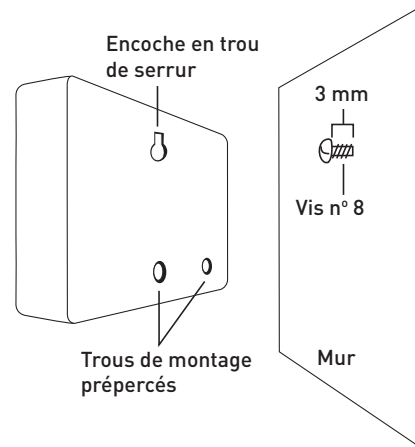
Figure 2 : Accrochez la minuterie au mur en insérant la vis dans l'encoche en trou de serrure
