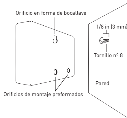
Figura 2: Cuelgue el temporizador en el tornillo. Para ello, use el orificio en forma de cerradura.
