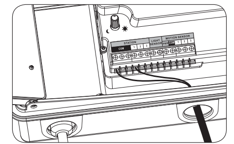
Figura 4: Conexión de los cables de alimentación a los terminales
