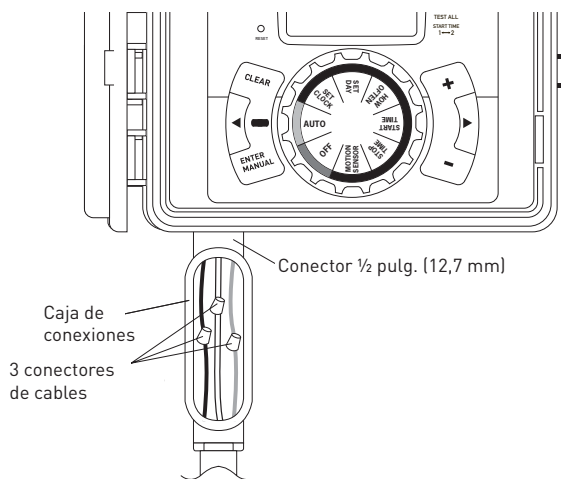
Figura 5: Uso de una caja de unión
