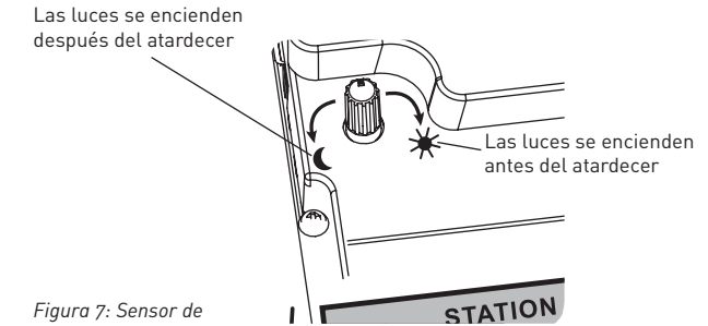
Figura 7: Sensor de iluminación Selector de ajuste
