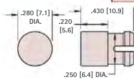
FIG. 2 T-1 3/4
