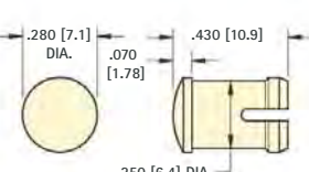
FIG. 4 T-1 3/4
