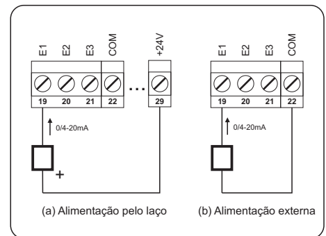
Ligação de sensor com saída em corrente
