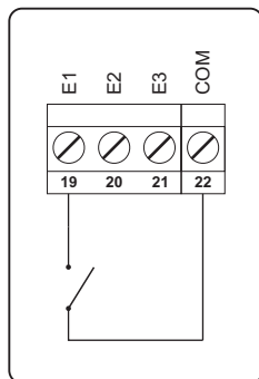
Ligação de contato seco
