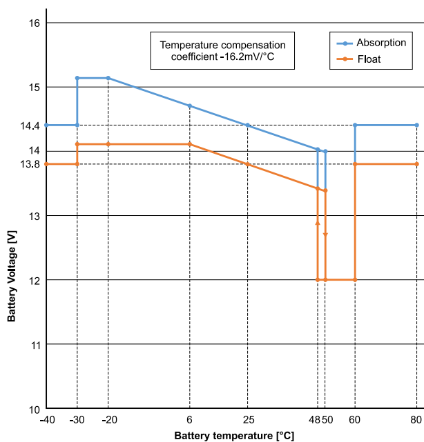
Temperatuurcompenseerde laadgrafiek
