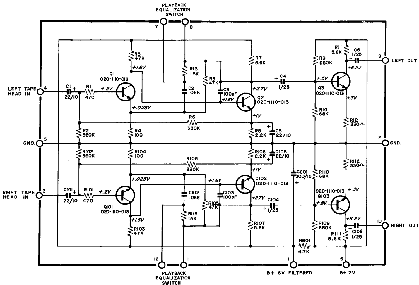
PC BOARD 019-1107-082 Rev.0
