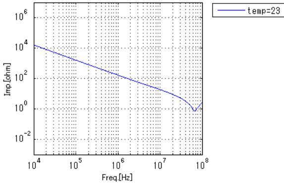
Cap.Freq.
