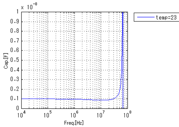
Cap.Freq.
