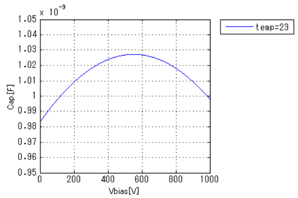
Cap.Vbias
