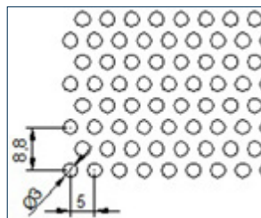
R3T5 Área Perforada 32,7%
