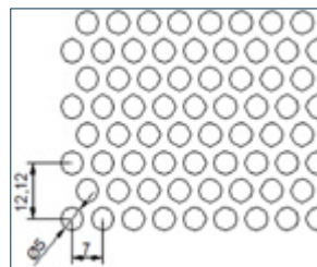
R5T7 Área Perforada 46,3%
