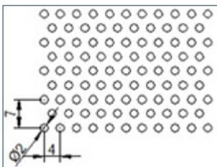
R2T4 Área Perforada 22,7%
