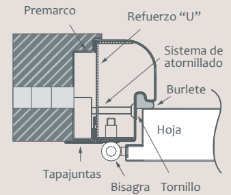
Montaje marco CR8 con premarco y tapajuntas
